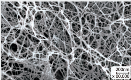
電子顕微鏡で観察したセルロースナノファイバー
