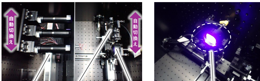
UV-LED 光源 紫外線放射照度計 放射照度標準受光器
