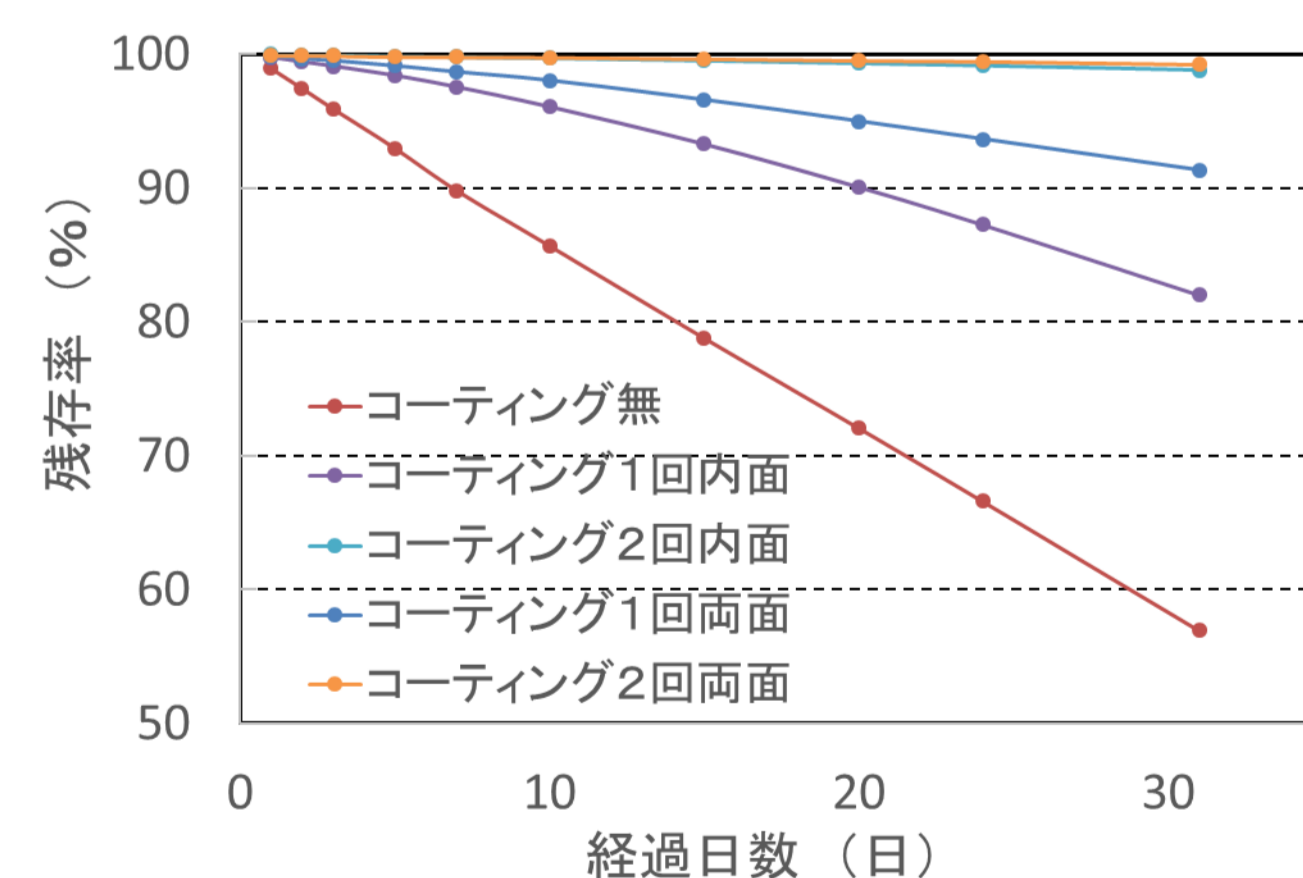
図3 模擬焼酎溶液の残存率経時変化
