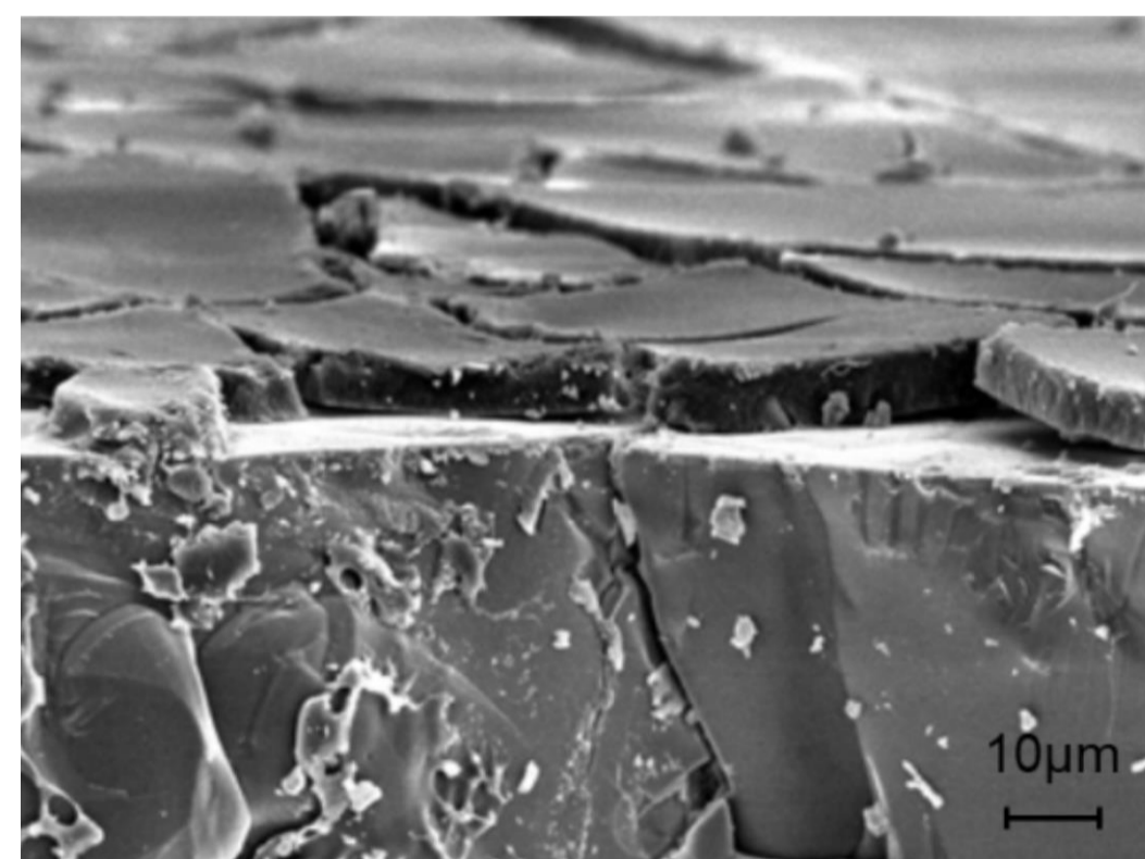
図2 缶内面塗料のSEM写真
