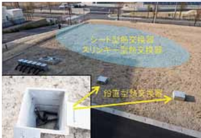
FREA地中熱利用システム実証試験場
