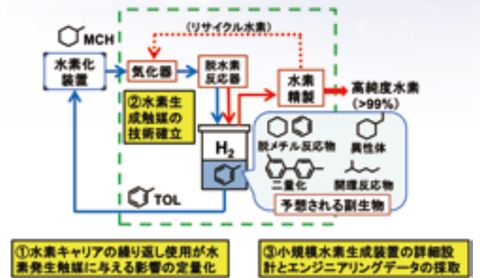
図1 MCHの水素化・脱水素循環
