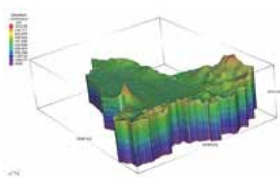
図1 津軽平野3次元地下水流動・熱輸送モデル
