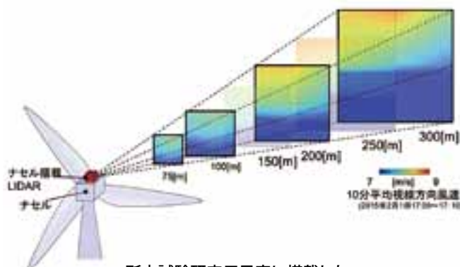
所内試験研究用風車に搭載した ナセル搭載LIDARの計測事例（視線方向風速分布） ※LIDAR: Light Detection and Ranging （レーザ光によって風向・風速をリモート計測する装置）の略
