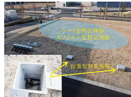
FREA地中熱利用システム実証試験場 深度1~2mの地下に設置するシート型熱交換器とスリッキー型熱交換器および深さ約40mの鉛直型(ボアホール型)の熱交換器を利用した地中熱システムです。
