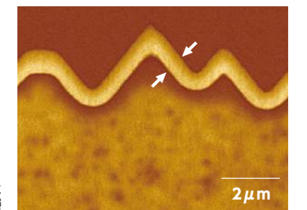
イオン注入により形成されたリン拡散層
