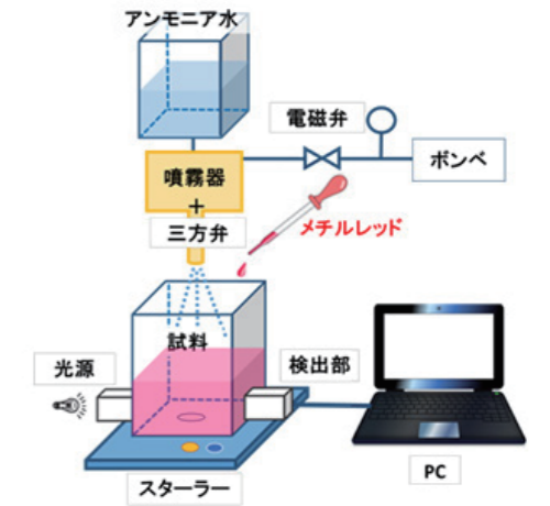
pH 自動調整装置の原理図 (色素の吸光度と pH 値の相関性を利用し、吸光度の変化をモニタしながら、アルカリ液の添加量を精密に制御して、溶液の pH を目的値まで正確に自動調整)
