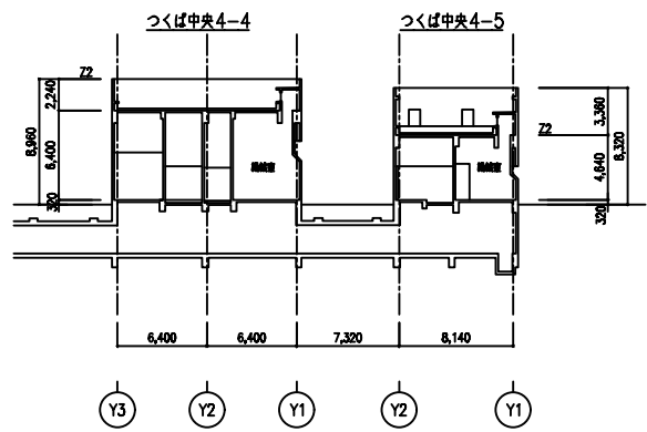
A - A' 断面図 S=1:200
