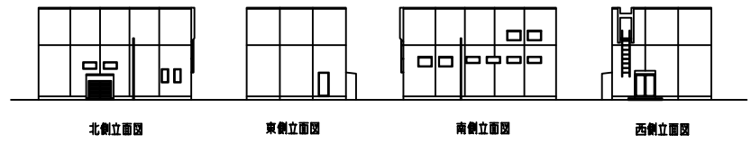
つくば中央4-5 S=1:200
