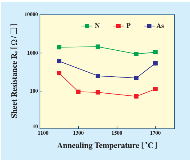
図6 R_s に対する活性化アニール温度依存性
